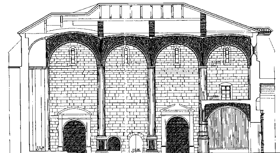
Secciones del templo parroquial. Dibujos del delineante D. Pedro Domínguez Barrios (enero de 2001).
